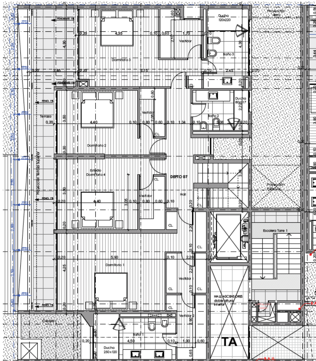
NIVEL +2
