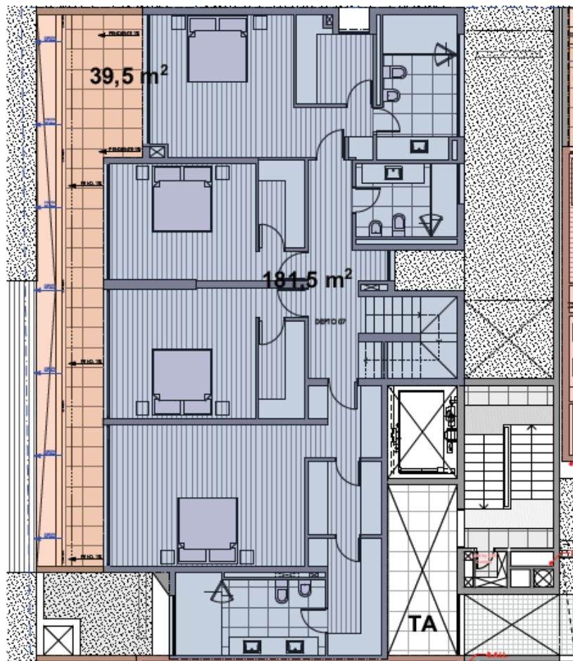
SUPERFICIES PISO 2
