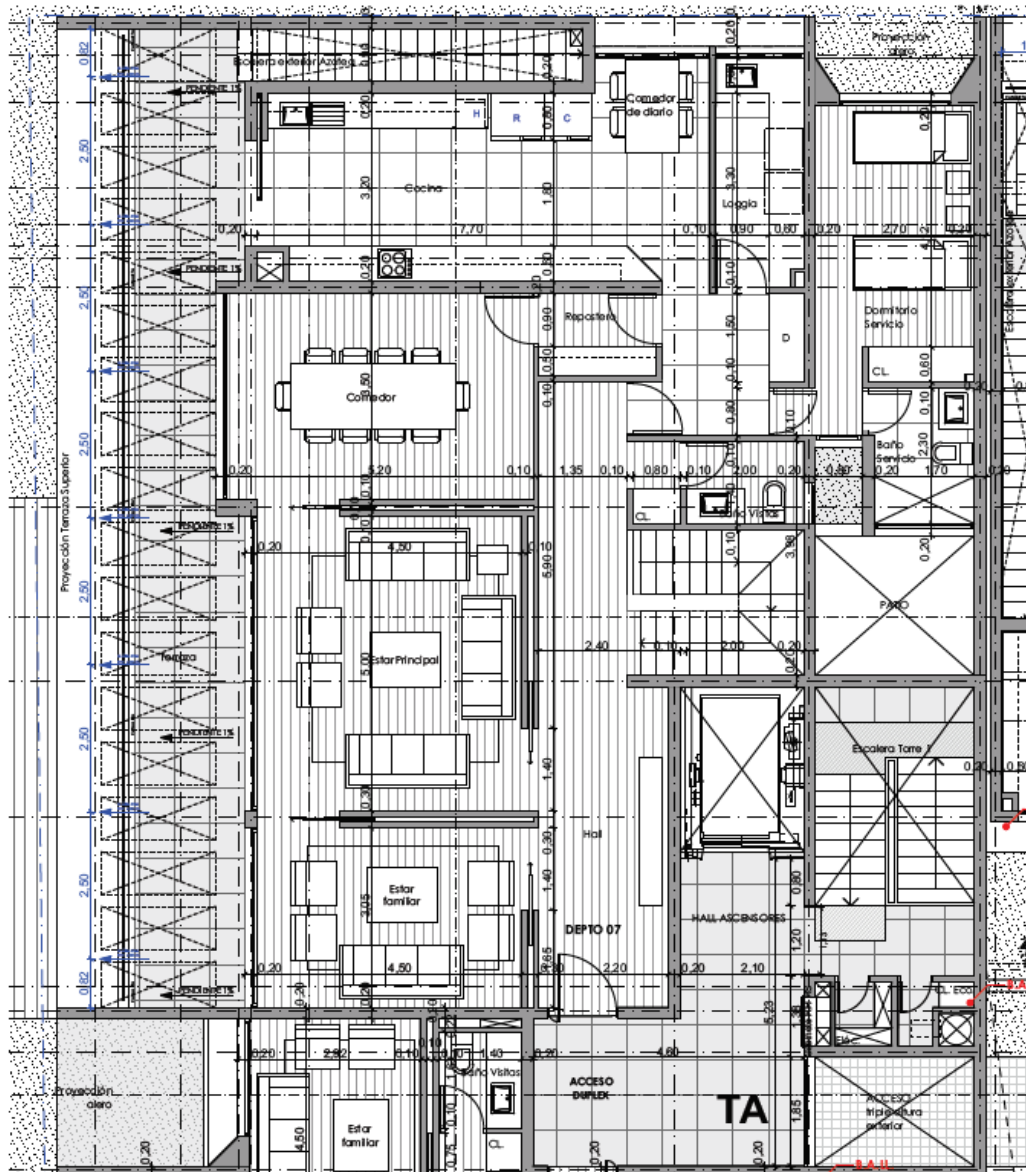
NIVEL +3 / ACCESO DEPTO. TIPO 7 (T1) DUPLEX / E.1:75
